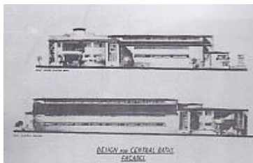
Angliai fürdőkomplexum terve
